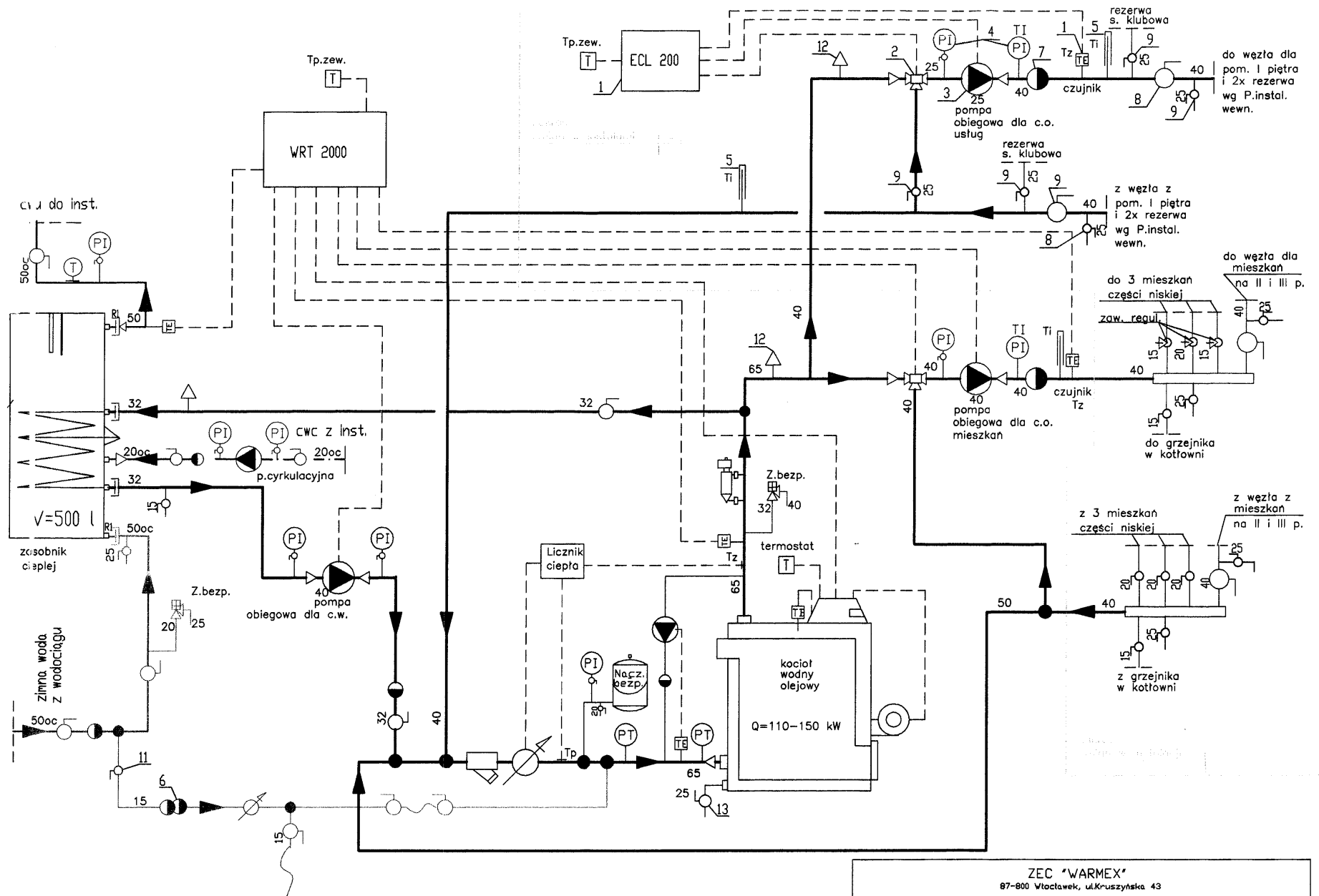
Schemat technologiczny
