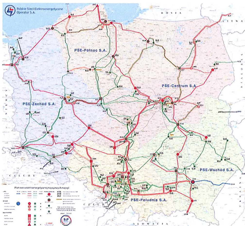
Rys. 16. Plan sieci elektroenergetycznej najwyższych napięć źródło: PSE
