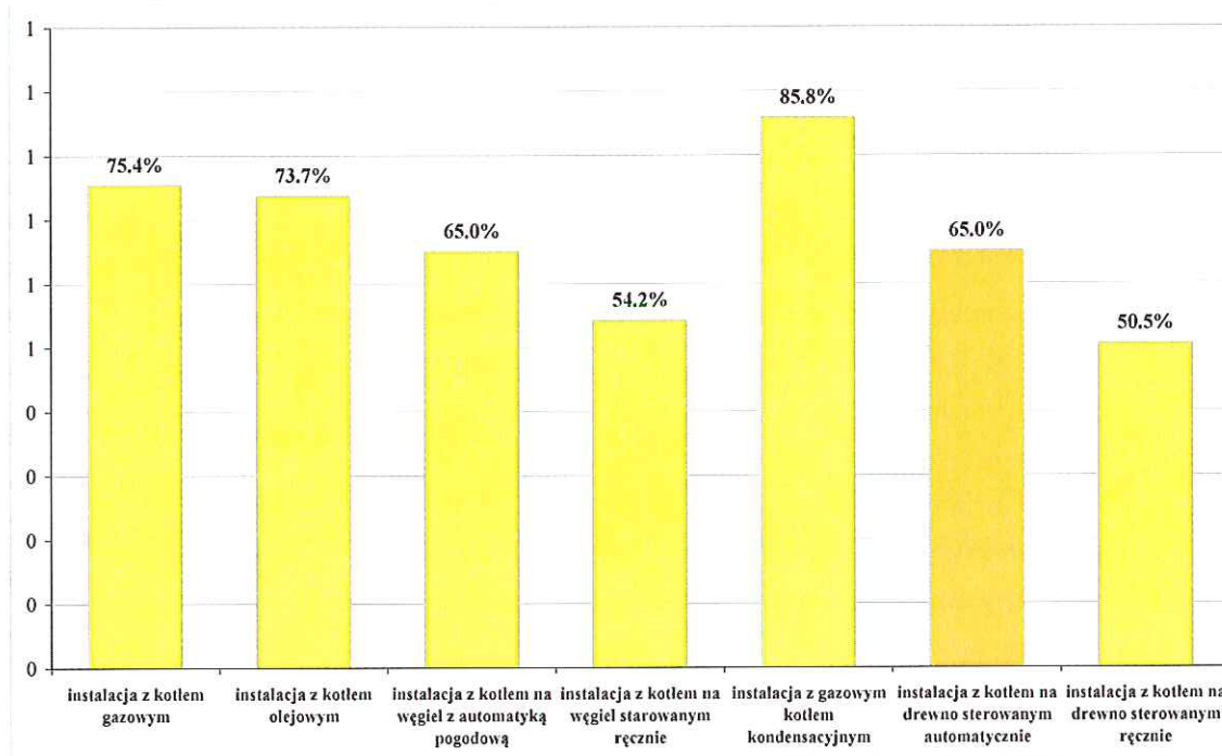
Rys. 13. Sprawność nowej instalacji c.o. wykorzystującej różne sposoby produkcji ciepła źródło: Dolnośląska Agencja Energii i Środowiska
