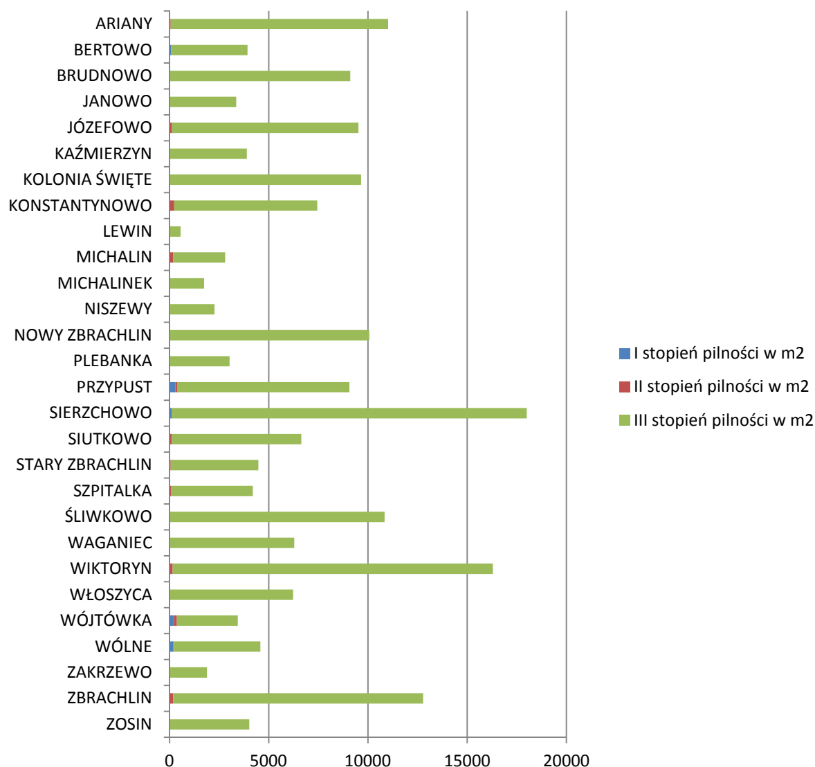
Wykres 3. Ilość azbestu i wyrobów zawierających azbest w m 2 wg poszczególnych kategorii stopnia pilności wymiany w poszczególnych miejscowościach Gminy Waganiec
